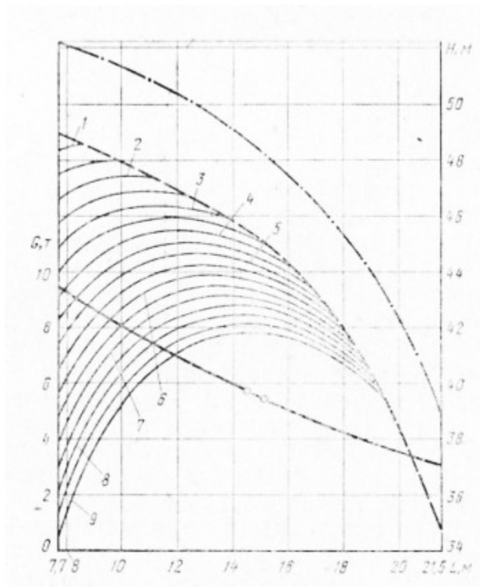
Рис. 20. МКГ-40 БСО 30,8—20 м
