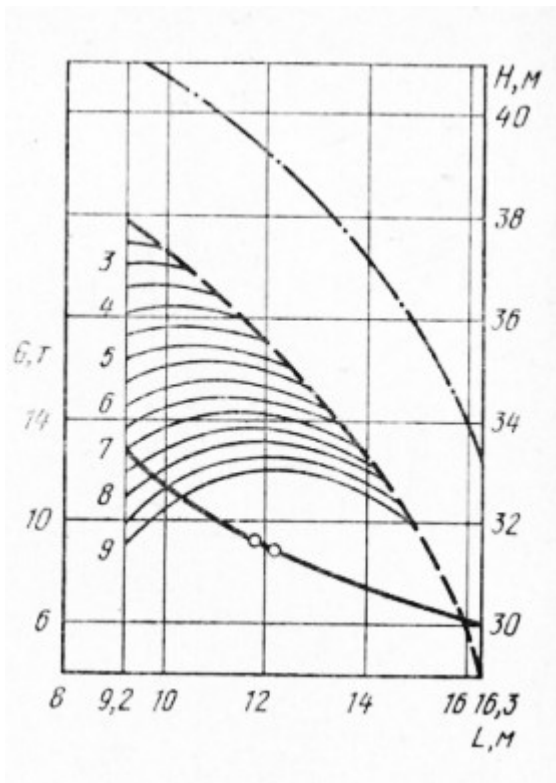
Рис. 17. МКГ-40 БСО 25,8—15 м
