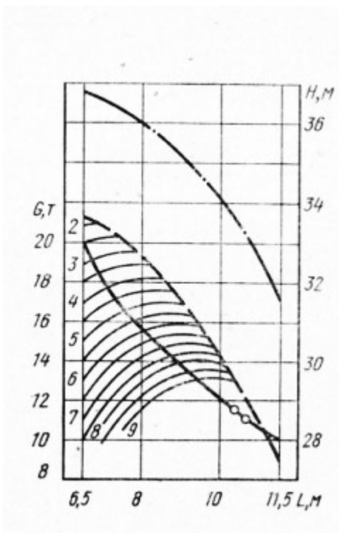
Рис. 16. МКГ-40 БСО 25,8—10 м
