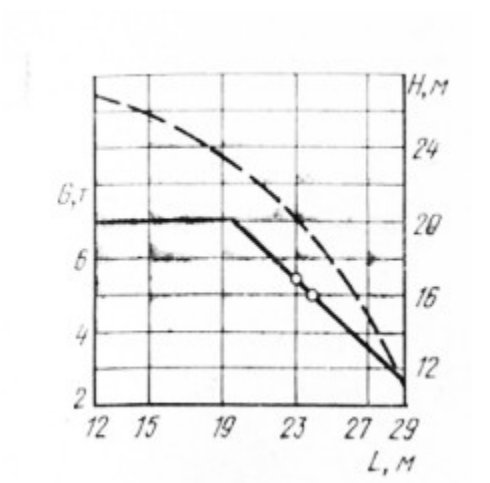
Рис. 10. МКГ-40 ВП стрела 25,8— 6 м
