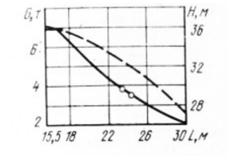
Рис. 12. МКГ-40 ВП стрела 35,8— в м
