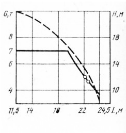
Рис. 9. МКГ-40 ВП стрела 20,8— 6 м
