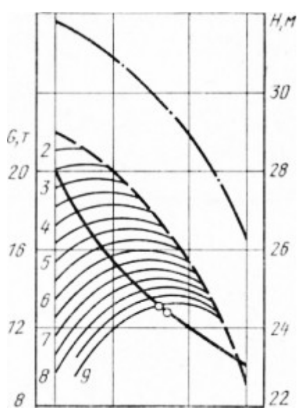
Рис. 14. МКГ-40 БСО 20,8—10 м
