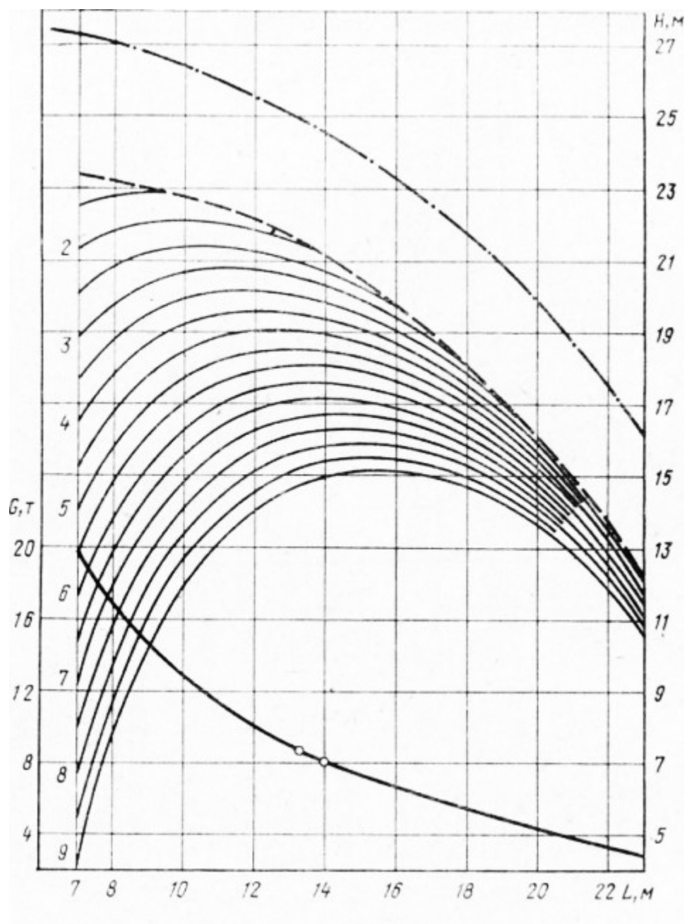
Рис. 5. МКГ-40 ОП стрела 25,8 6 м
