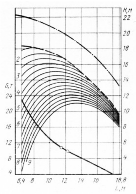
Рис. 4. МКГ-40 ОП стрела 20,8— 6 м
