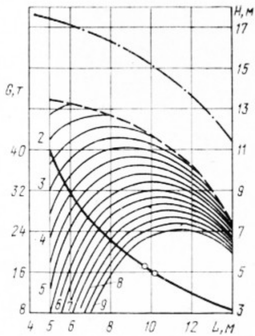
Рис. 3. МКГ-40 ОП стрела 15.8— 6 м
