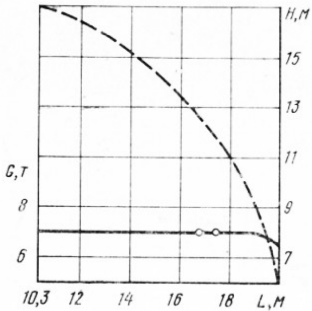
Рис. 8. МКГ-40 ВП стрела 15,8—6 м
