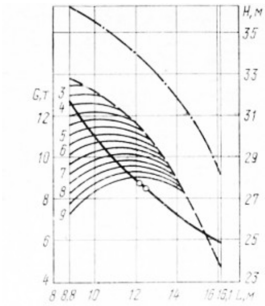
Рис. 15. МКГ-40 БСО ,20.8—15 м
