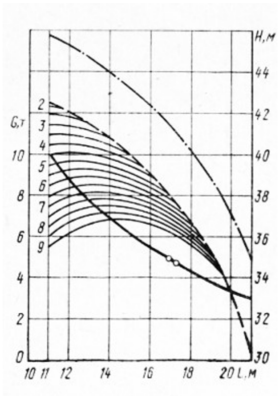
Рис. 18. МКГ-40 БСО 25,8—20 м
