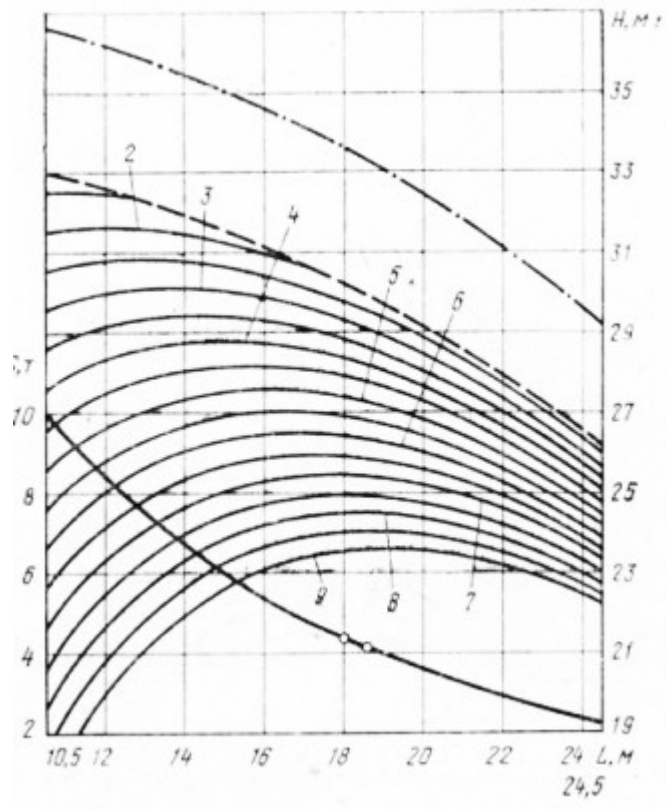
Рис. 7. МКГ-40 ОП стрела 35,8—6 м
