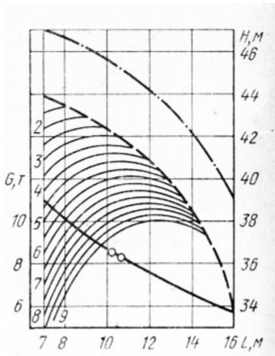
Рис. 19. МКГ-40 БСО 30,8—15 м
