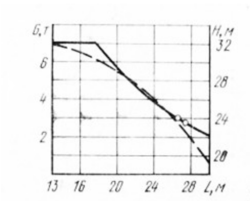
Рис. 11. МКГ-40 ВП стрела 30,8— 6 м
