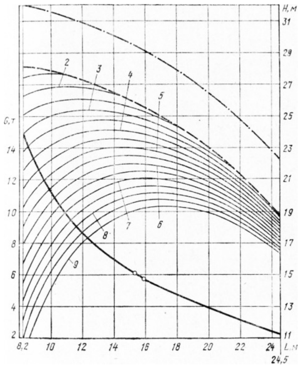
Рис. 6. МКГ-40 ОП стрела 30,8—6 и
