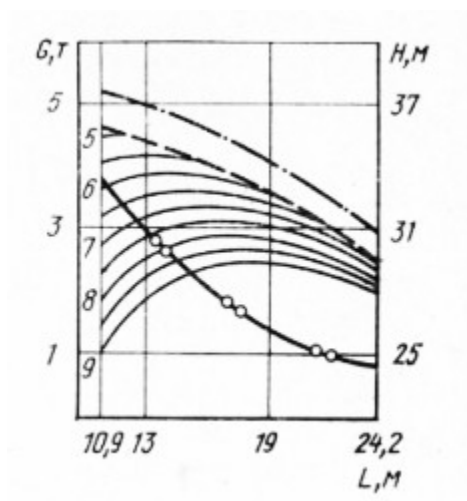
Рис. 1. ДЭК-251 ВП стрела 32,75—5 м
