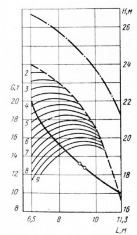
Рис. 13. МКГ-40 БСО 15,8—10 м
